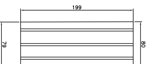
Silka E8 Widok z boku Skala 1:4
